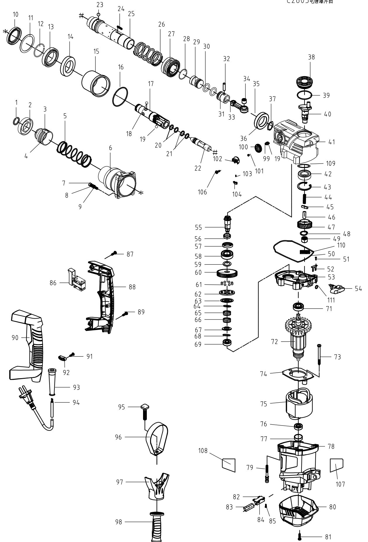
C2803电锤爆炸图
